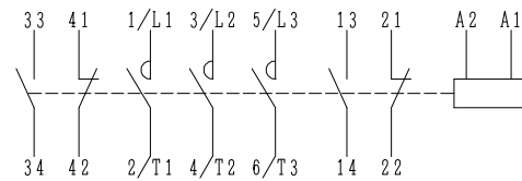
AUX. CONTACTS : 2 a 2 b CONTACTS ARRANGEMENT.
