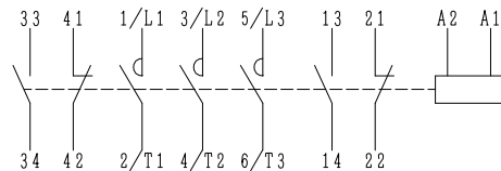
AUX. CONTACTS. : 2a2b CONTACTS ARRANGEMENT.
