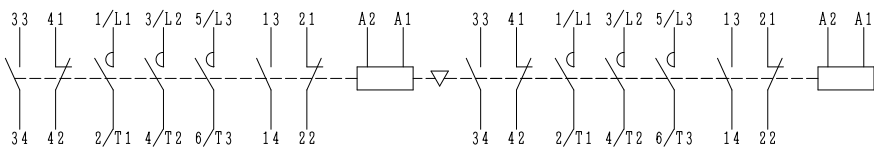
AUX. CONTACTS : 2a2b x 2 CONTACTS ARRANGEMENT.
