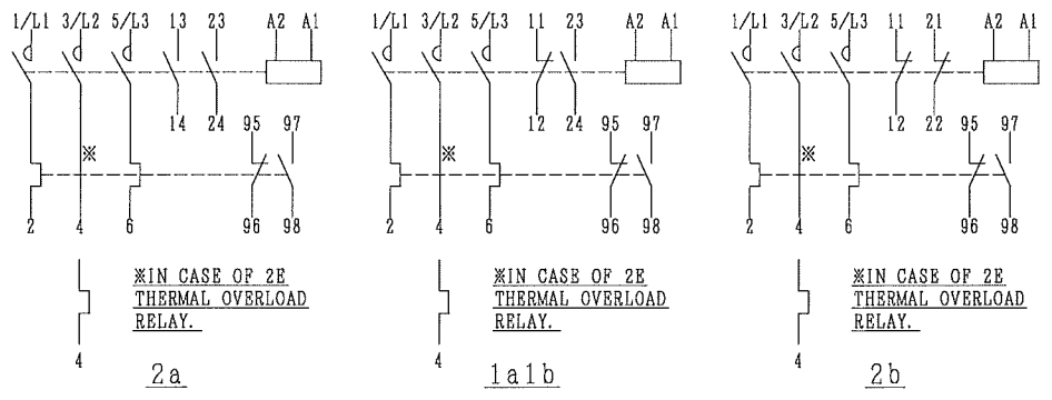
AUX. CONTACTS CONTACTS ARRANGEMENT.
